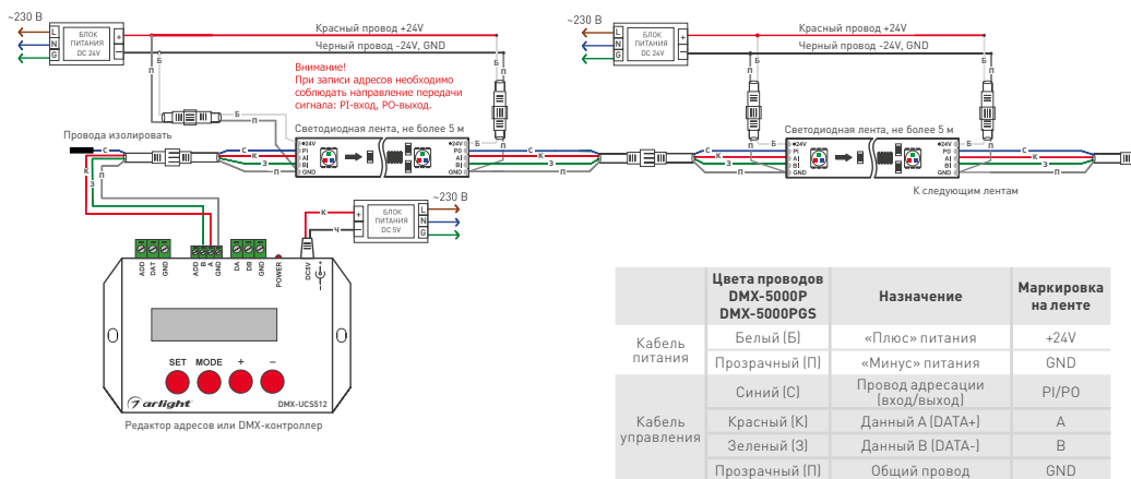
Рисунок 2. Схема подключения лент DMX-5000P и DMX-5000PGS на примере редактора адресов DMX-UCS512 и с использованием отдельных блоков питания
